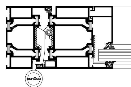
Horizontalschnitt Schüco Tür ADS 80 FR 30, Maßstab 1:3 Horizontal section detail, Schüco Door ADS 80 FR 30, scale 1:3
